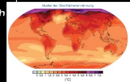
Projizierte Änderungen der Erdoberflächentemperatur für das spätere 21. Jahrhundert (2090-2099) gemittelt aus verschiedenen Szenarien in Bezug zum Zeitraum 1980-1999.
