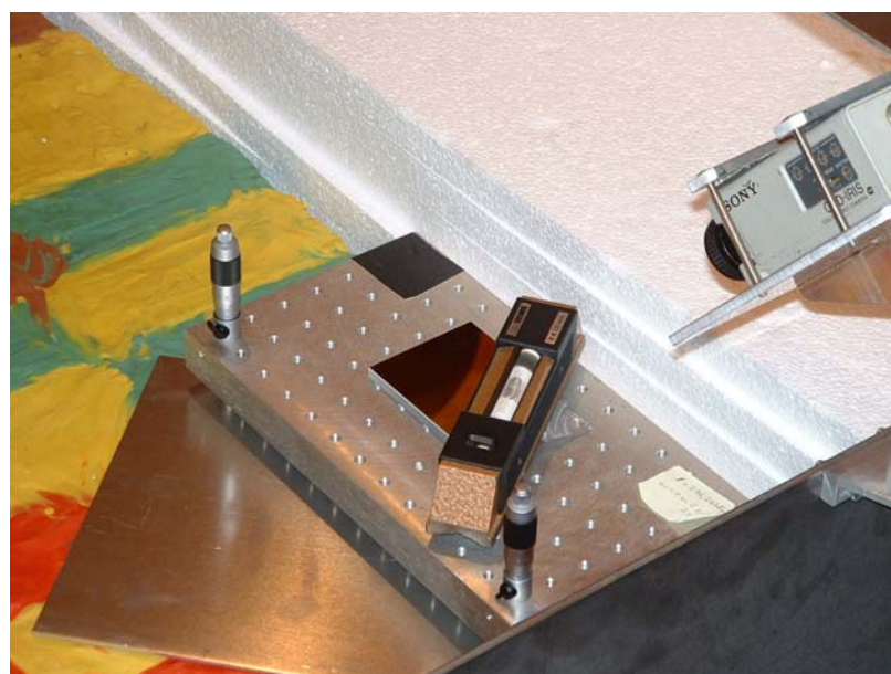
Die Präzisionswasserwaage liegt auf einem Metallbrett, welches durch die beiden Stellschrauben an den Seiten exakt waagrecht ausgerichtet werden kann.
